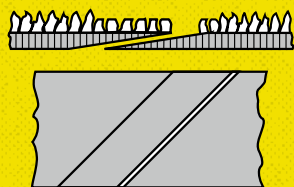
Forma 2 Połączenie ukośne, zakładkowe, klejone. Zeszlifowane wierzchołki ziaren w celu zapewnienia spokojnego biegu pasa
