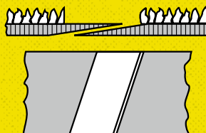
Forma 5 Połączenie zakładkowe. W miejscu połączenia ziarno w pełni zeszlifowane. Umożliwia spokojne (bezударowe) przejście połączenia przez strefę szlifowania. Zastosowanie w połączeniu z płaską stopą dociskową.
