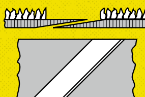
Forma 5 Połączenie ukośne, zakładkowe, klejone. W miejscu połączenia ziarno w pełni zeszlifowane. Preferowane połączenie w obróbce drewna z profilową stopą dociskową
