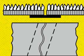
Forma 7 G Połączenie sinusoidalne, podklejone folią wzmocnioną płótnem. Zapewnia bieg taśmy bez uderzeń; do obróbki kruchych elementów, spełniające wysokie wymagania.
