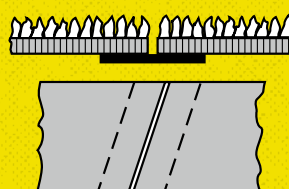
Forma 4 G Połączenie ukośne. Połączenie stykowe podklejone folią wzmacnianą płótnem. Standardowe połączenie dla pasów poliestrowych. Wysoka odporność na rozrywanie.
