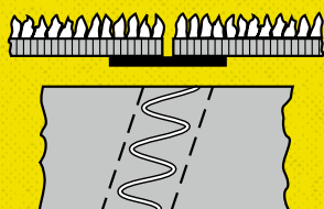
Forma 3 G Połączenie w zygzak, podklejone folią wzmocnioną płótnem. Zapewnia bieg taśmy bez uderzeń; do obróbki kruchych elementów, głównie szkła.
