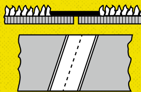
Forma 6 G Połączenie ukośne. Połączenie stykowe, podklejone po stronie ziarna folią wzmocnioną płótnem. W miejscu połączenia ziarno w pełni zeszlifowane. Zastosowanie w połączeniu z płaską stopą dociskową.
