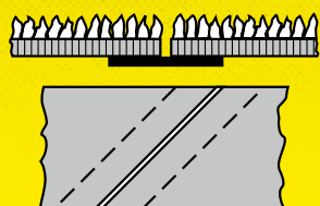
Forma 4 G Połączenie ukośne. Połączenie stykowe, podklejone folią wzmocnioną płótnem. Nadaje się do pracy na taśmie wolnej, do obróbki spełniającej wysokie wymagania.
